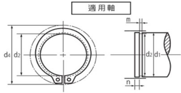
d4為固定環安裝至d1時外周的最大直徑 (間隙外徑)
