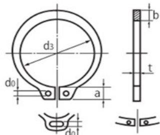
尺寸No.9以下 尺寸No.170以上
