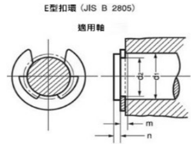
E型固定環 (E型扣環) 尺寸圖
