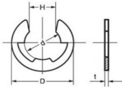
E型固定環 (E型扣環) 尺寸圖
